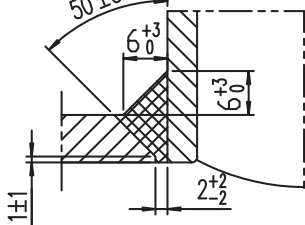
D1,D2,D3,D4 焊接详图 Welding detail of D1,D2,D3,D4 NO SCALE
